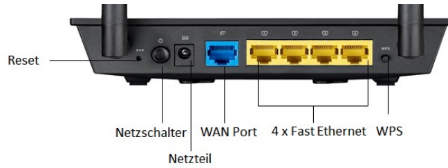
Ansicht Router-Anschlüsse Rückseite:
