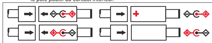
Fig.9: Ajuster la polarité
