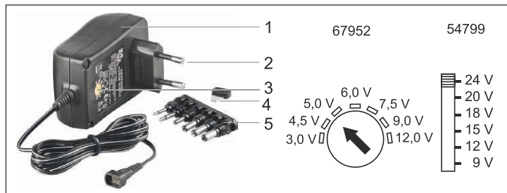
Fig.8: Eléments de commande
