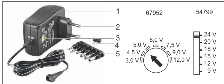
Fig.11: Elementi di comando
