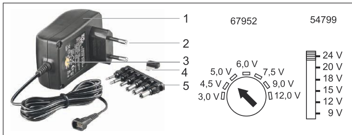
Fig.2: Bedienelemente
