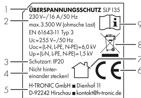
Bild 1 Typenschild
