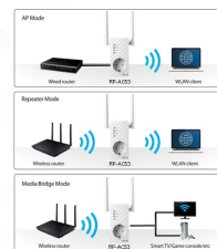
3-in-1 Repeater, AP und Mediabridge
