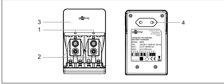
Fig.14: Fişli şarj cihazı
