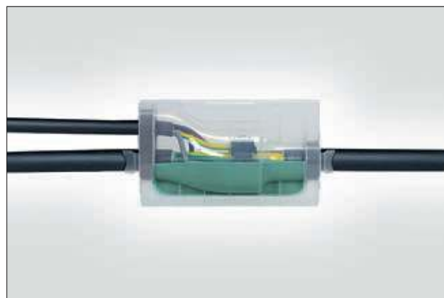
Parallelabzweiggarntur PAH-4 140/420, Hausanschlussgarntur.
