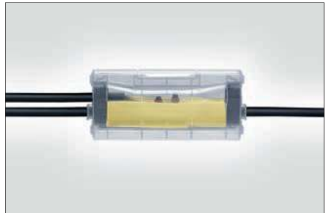
Parallelabzweiggarnitur PA-11 58/230.
