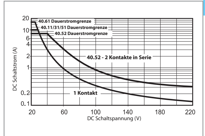
H 40.2 - Gleichstromschaltvermögen bei DC1 - Belastung Typ 40.31/51/52/61 (Seite 4) und 40.11 (Seite 5)
