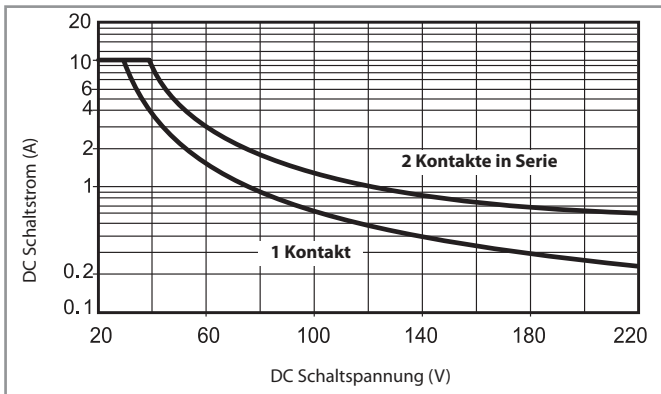
H 40.6 - Gleichstromschaltvermögen bei DC1 - Belastung Typ 40.62 (Seite 5)
