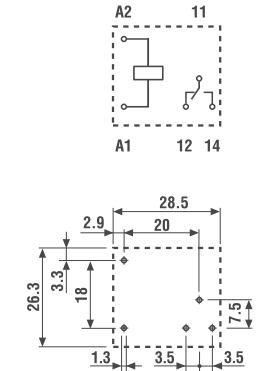
Ansicht auf die Anschlüsse 3.5 mm Pinlänge für Leiterplatte
