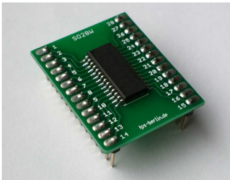
Anwendungsbeispiel Adapterplatine SO28W - SO28X
