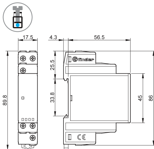
Type 70.61 Schraubklemmen
