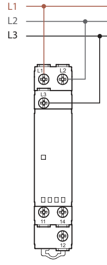
Typ 70.61
