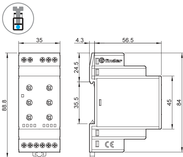
Type 70.51 Schraubklemmen
