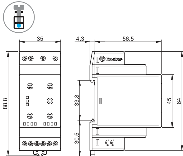
Typ 70.42 Schraubklemmen
