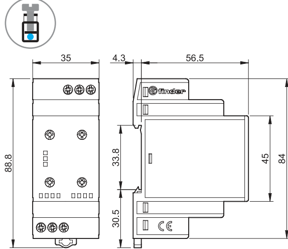
Typ 70.31 Schraubklemmen
