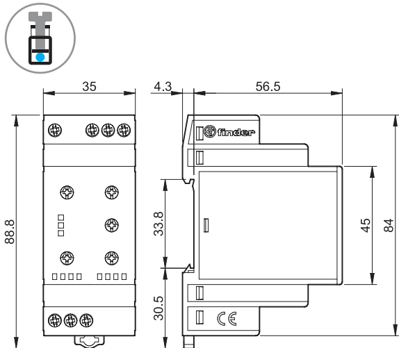
Typ 70.41 Schraubklemmen
