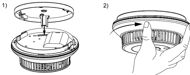
Abbildung 11: Rauchwarnmelder einrasten
