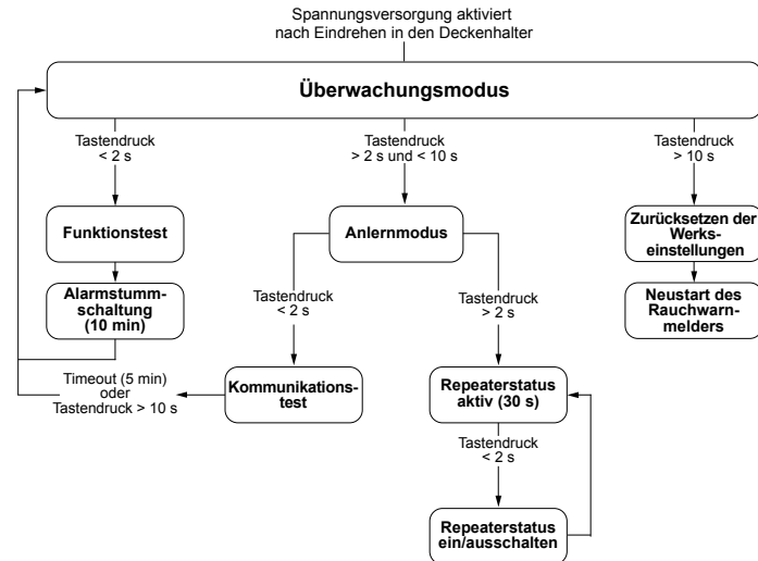
Abbildung 13: Bedienstruktur Rauchwarnmelder
