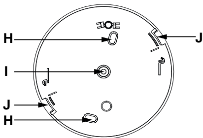
Abbildung 3: Deckenhalter
