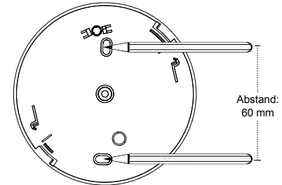
Abbildung 12: Markierung zwei Bohrlöcher
