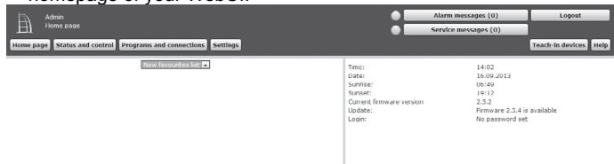
Fig. 5: WebUI homepage
