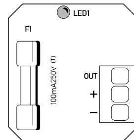
Bild 3 Layout für den elektrischen Anschluss
