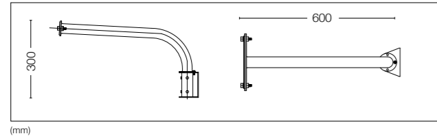
WANDHALTERUNG - ABMESSUNGEN
