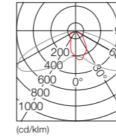
LICHTVERTEILUNG
