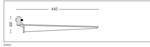
BODENHALTERUNG - ABMESSUNGEN
