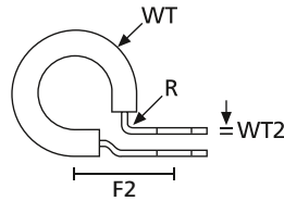
Aluminiumschelle mit Chloroprenschutzprofil (Seitenansicht)
