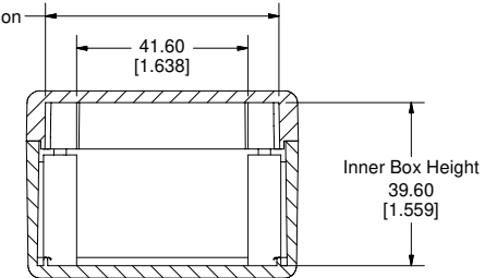
SECTION D-D SCALE 1 : 1
