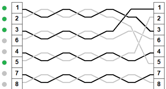
Fig. 5 Verdrahtungsfehler
