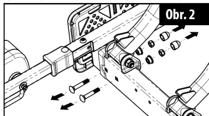
Obrázek 4: Demontáž upevňovacích šroubů
