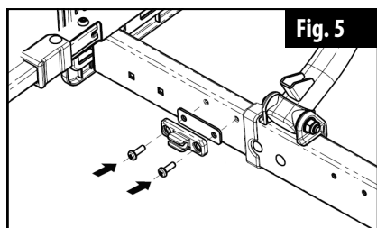
Figura 7: Montaggio delle graffe di fissaggio
