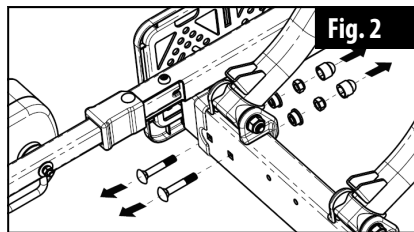
Figura 4: Rimozione delle viti di fissaggio
