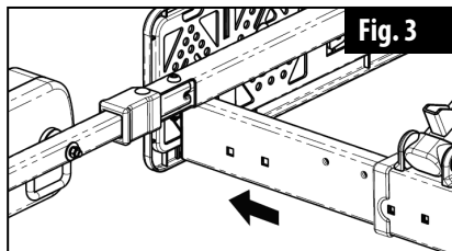
Bild 5: Herausziehen der Rahmenverlängerung
