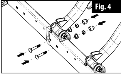
Bild 6: Einsetzen der Halteschrauben
