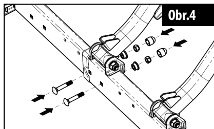
Obrázek 6: Vložení upevňovacích šroubů
