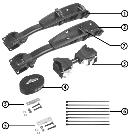
Obrázek 1: Rozsah dodávky
