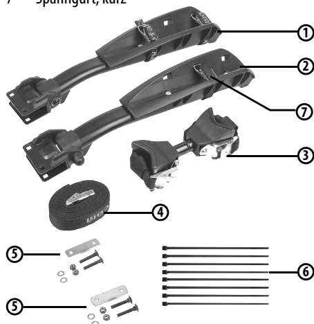
Bild 1: Lieferumfang
