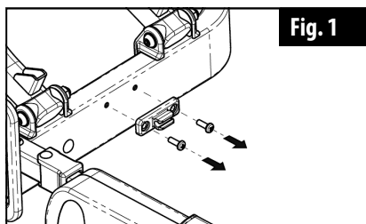
Bild 3: Entfernen der Halteklammern
