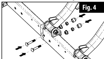
Figure 6 : Introduction des vis de retenue
