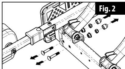
Bild 4: Entfernen der Halteschrauben
