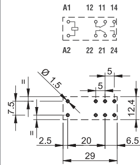
Ansicht auf die Anschlüsse 5.3 mm Pinlänge für Leiterplatte oder Fassung Serie 95
