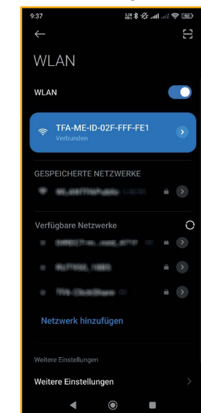
Beispiel Android
