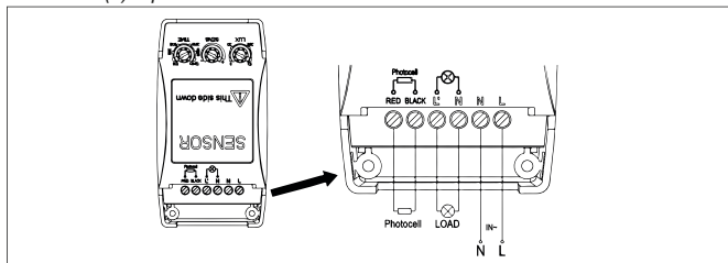
Fig.17: Installazione
