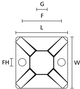
MB3-MB5 (Draufsicht)
