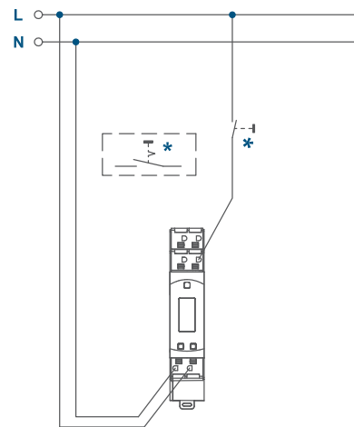
Anschluss von Tastern/Schaltern (Eingänge):
