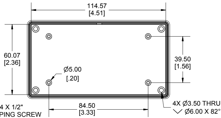
INSIDE LID
