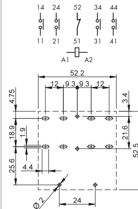
Ansicht auf die Anschlüsse
