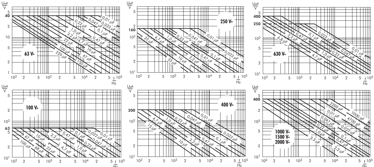
Wechselspannung in Abhängigkeit von der Frequenz bei 10° C Eigenwärmung (Richtwerte).
