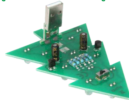
Platzierung des USB-Steckers für waagrenten USB-Ausgang:
