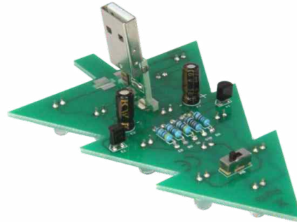
Platzierung des USB-Steckers für senkrechten USB-Ausgang:
