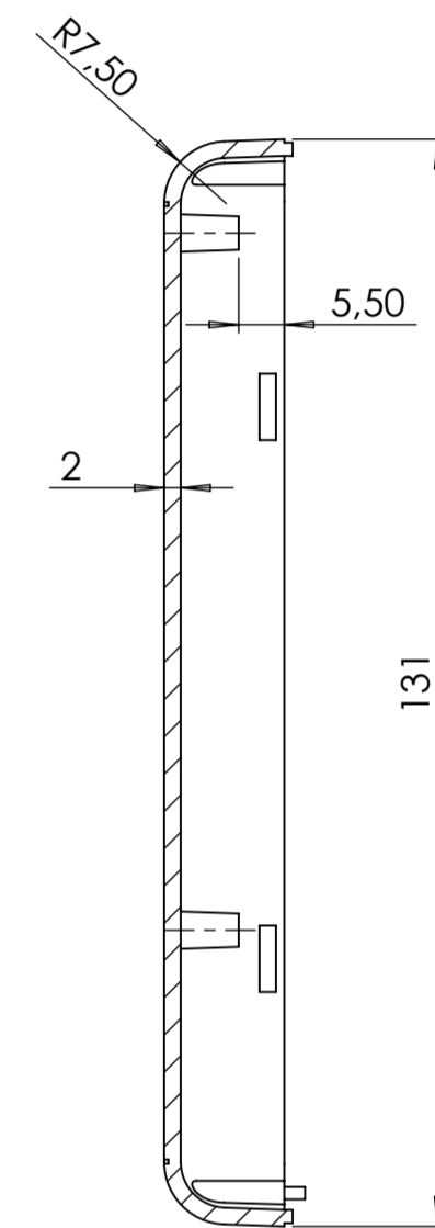
SEZIONE D-D
