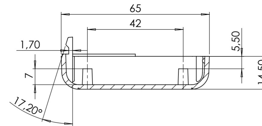
SEZIONE E-E
