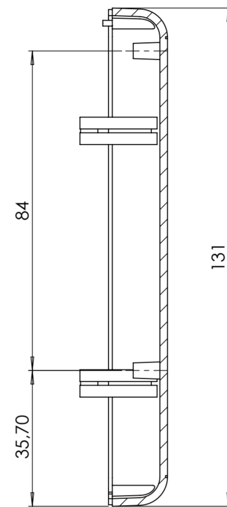
SEZIONE C-C
