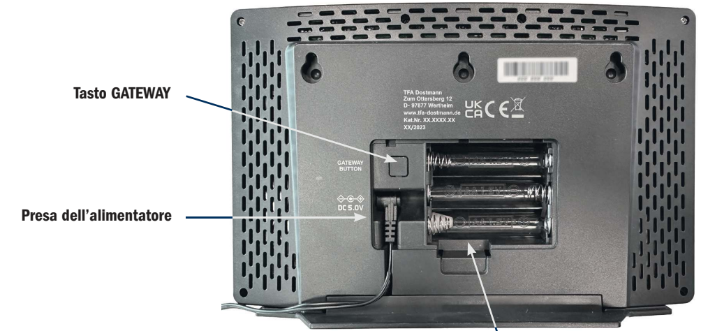
Tasto GATEWAY Presa dell'alimentatore Vano batteria
