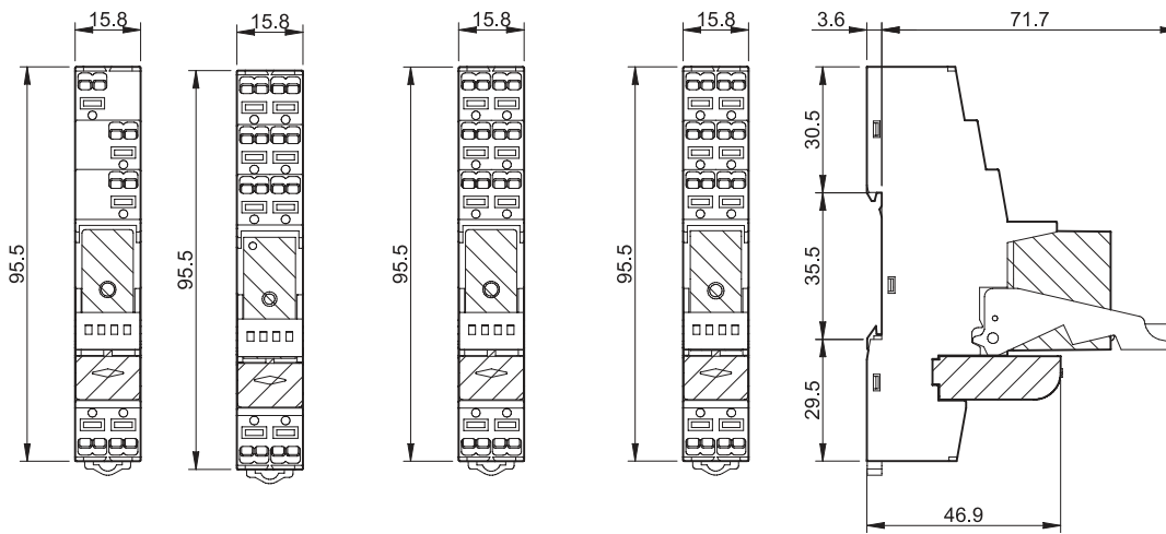
Typ 48.P3 Push-In - Klemmen
