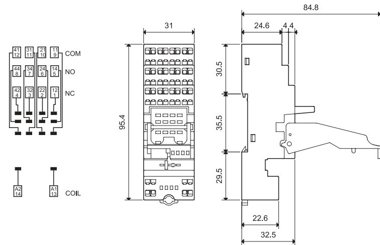
Fassung + Kammbrücke
