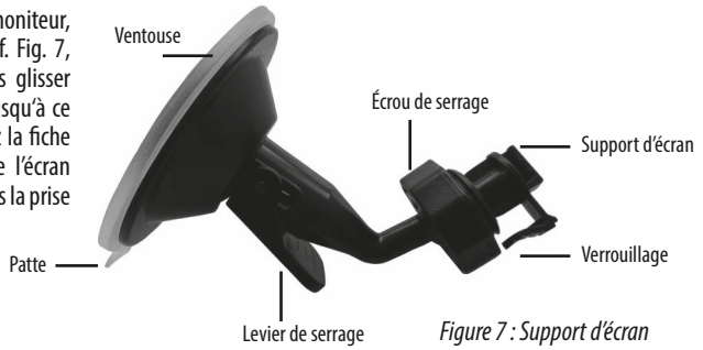
Figure 7 : Support d'écran
