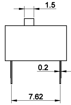
Extend actuator(E)
